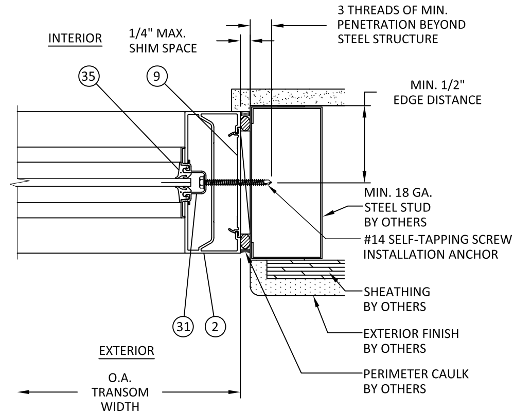
K 6 HORIZONTAL SECTION TRANSOM JAMB - STEEL STUD
